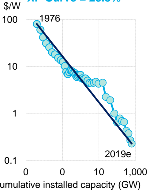
Solar module price ($/W)
