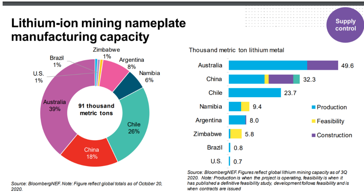
Figura 4: Capacidad mundial de extracción y recuperación de litio (tercer trimestre de 2020)
