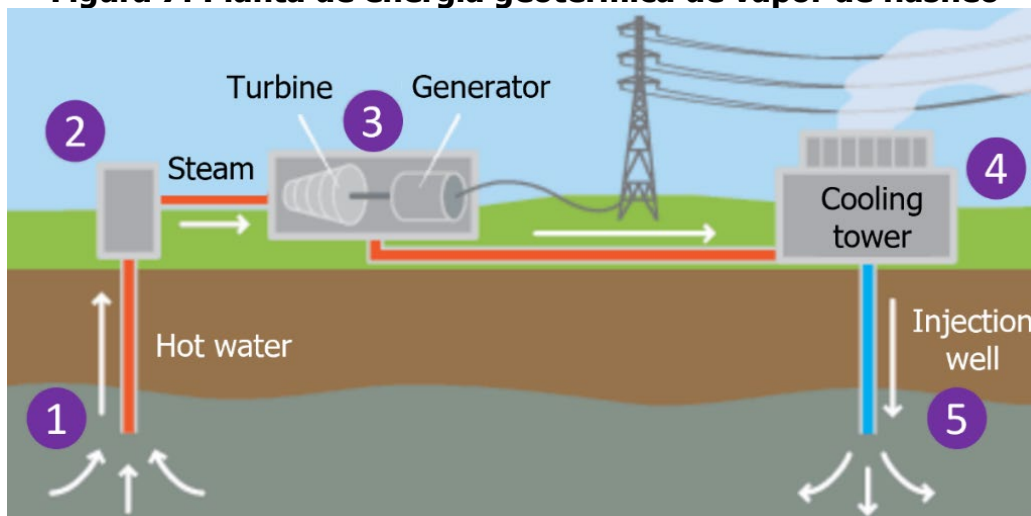
Figura 7: Planta de energía geotérmica de vapor de flasheo
